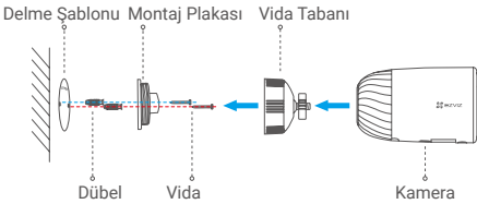
Şek.2 Vida Tabanı ile Monte Etme
